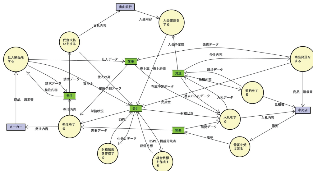
図 3 Clear-ERP の業務モデル (DFD 表記)
