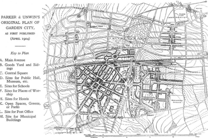
図 4：パーカーとアンウィンによるレッチワースのレイアウト（初出：1904 年春） 20
